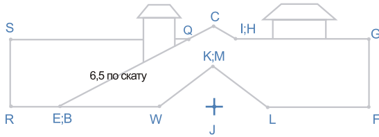
ВИД "С"
